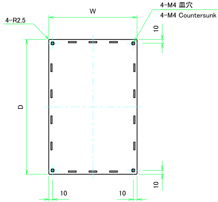
上カバー表面 / Top cover Frontside
