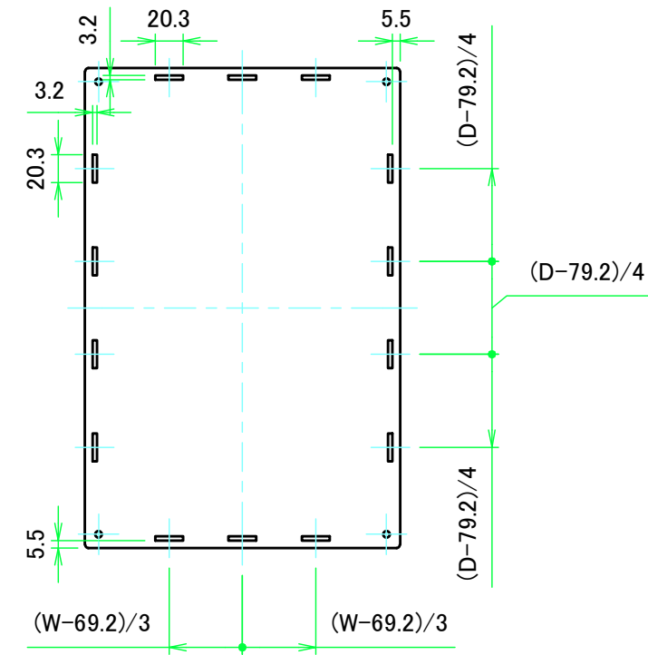
上カバー裏面 / Top cover Backside
